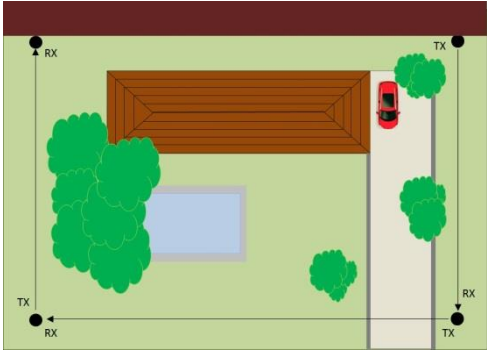
SOLUZIONE CON BARRIERE BIDIREZIONALI E TERMINALI
