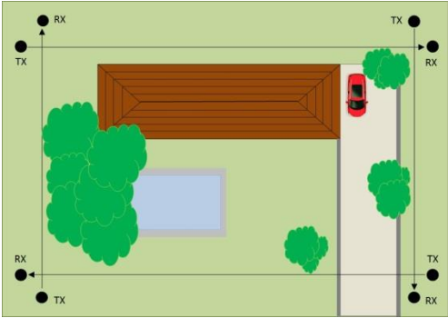
SOLUZIONE CON BARRIERE TERMINALI
